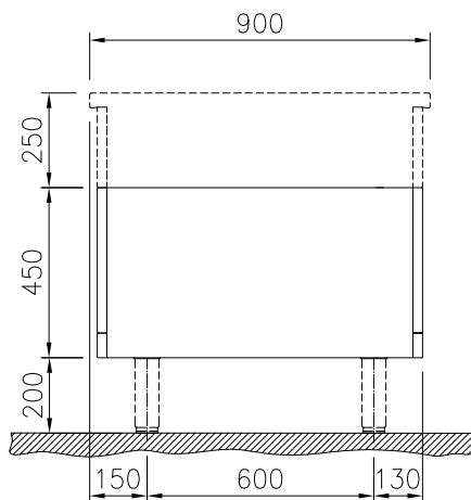
Zij aanzicht
