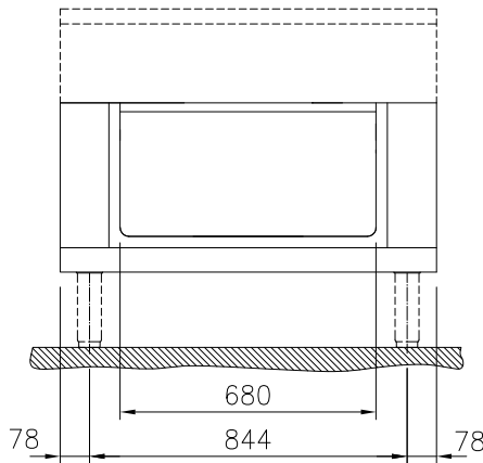
Front aanzicht
